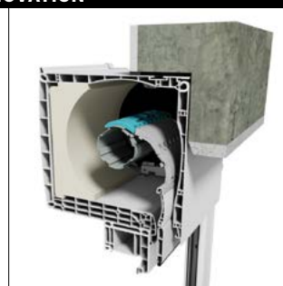
BLOC-BAIE RÉHABILITATION. POSE APRÈS DÉPOSE TOTALE
