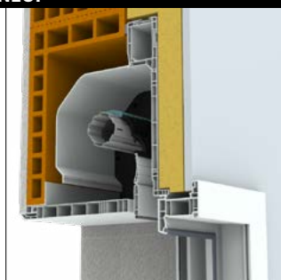
LA SOLUTION VOLET ROULANT POUR POSE SOUS DEMI-LINTEAU
